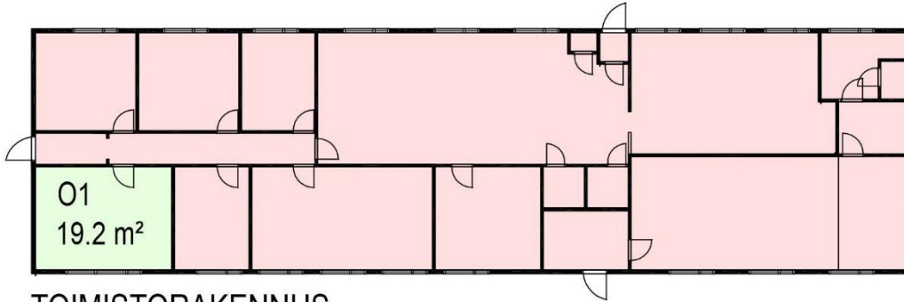
TOIMISTORAKENNUS
